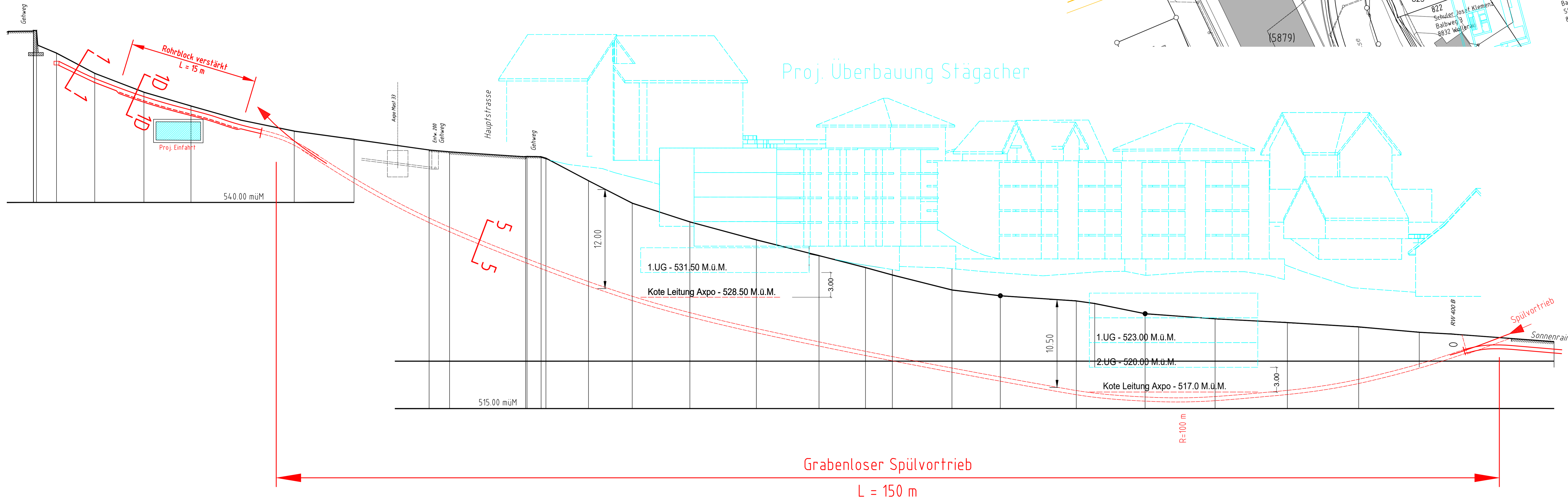
Längsschnitt D-D 1:200
